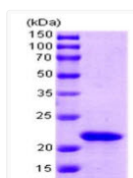
15% SDS-PAGE (3µg)
