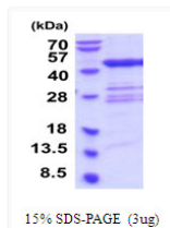
15% SDS-PAGE (3µg)
