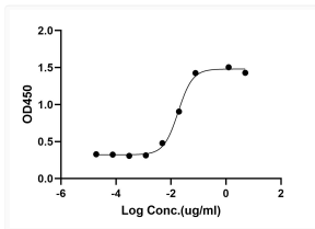
ELISA: STJA0038425
