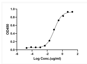
ELISA: STJA0038327
