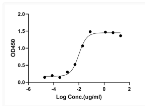
ELISA: STJA0038254
